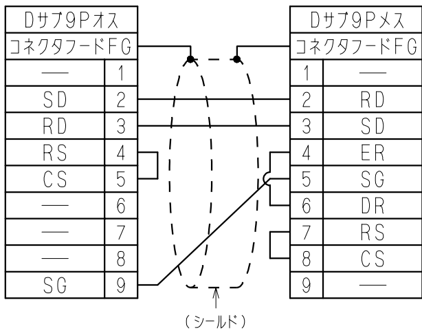
* 配線図
