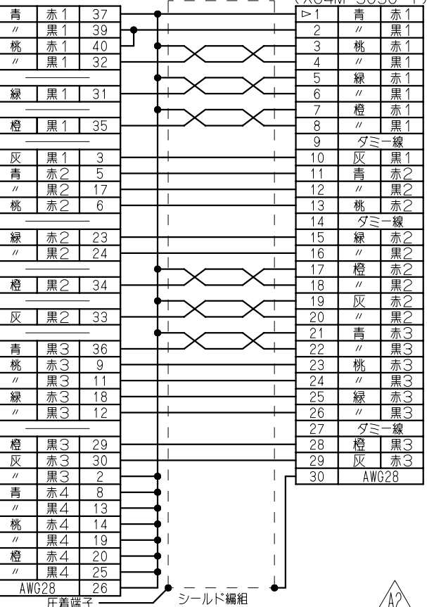
CJ1M-CPU22/23中継ユニット接続ケーブル (W系)
