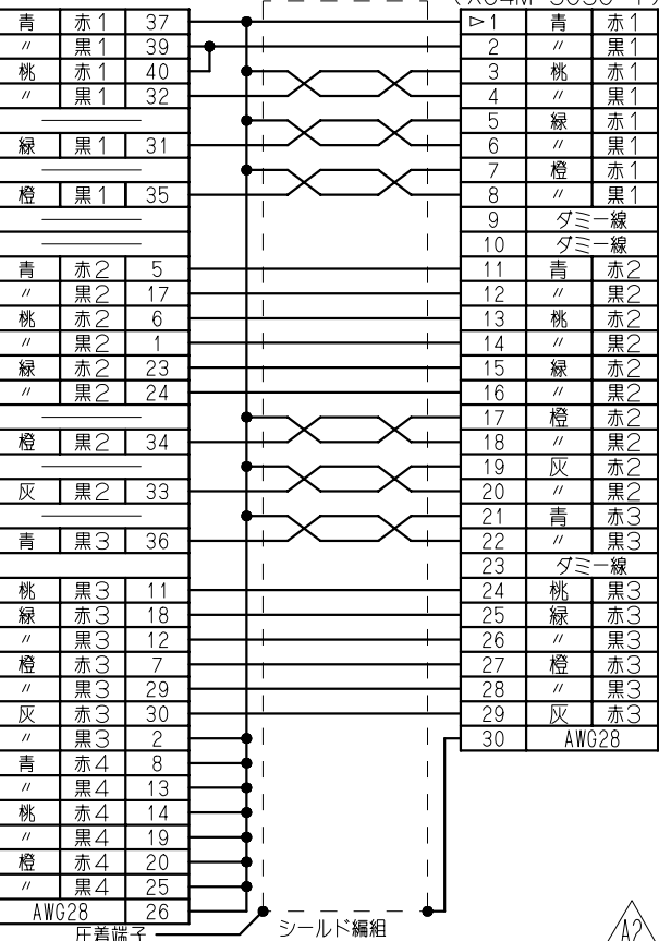
CJ1M-CPU22/23中継ユニット接続ケーブル (SS系)
