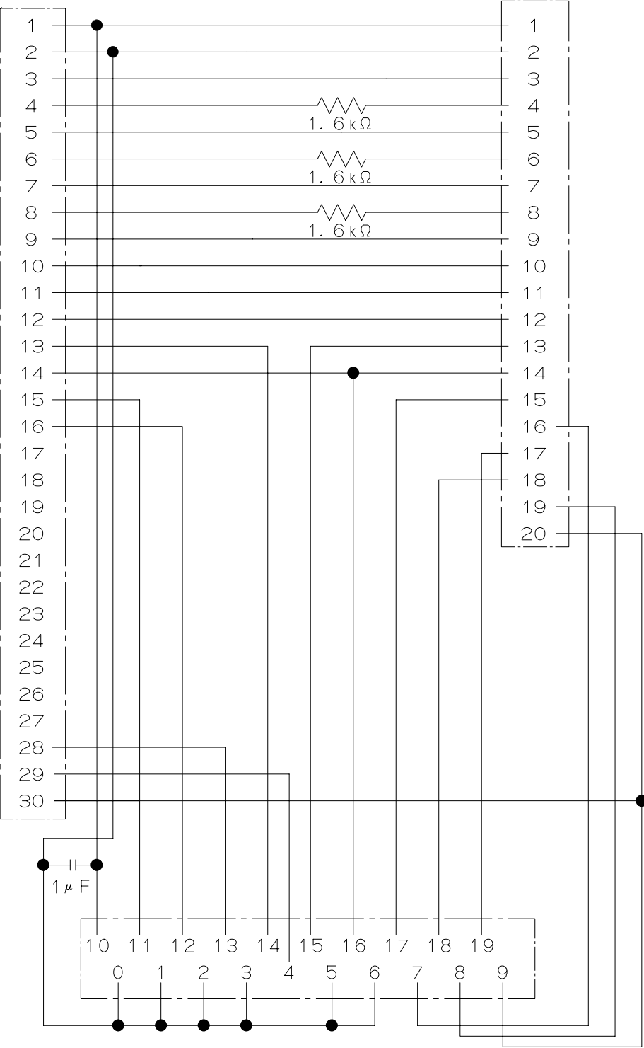
XG4A-3031 (PLC側)
