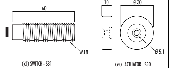
(d) SWITCH - S31 (e) ACTUATOR - S30
