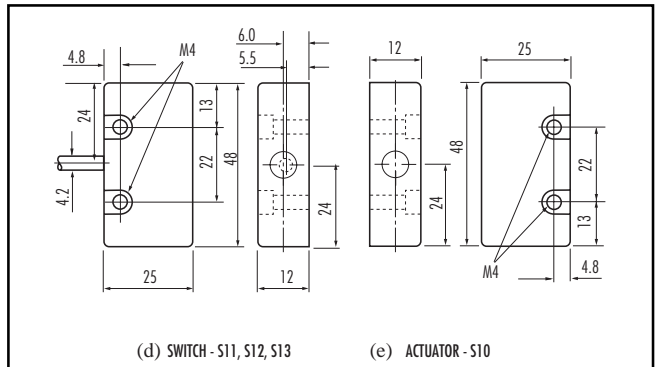
(d) SWITCH - S11, S12, S13 (e) ACTUATOR - S10
