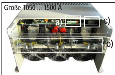
Abbildung 2.4.1: Klemmenlokalisierung
