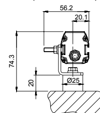
équerre de fixation standard + support anti-vibration (ST-K 4/6 AV)
