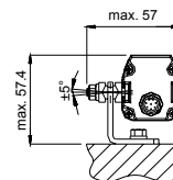
équerre de fixation standard + support orientable (ST-K 4/6 OR)
