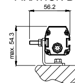
équerre de fixation standard ST-KSTD
