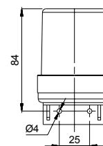
LMS-3 voyant d'inhibition
