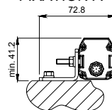
équerre de fixation standard ST-KSTD
