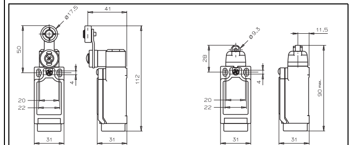
Fig. 2: Plan coté i10-R
