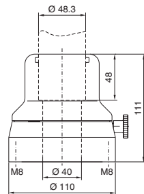
2 Fixation par l'avant CP 6663.400
