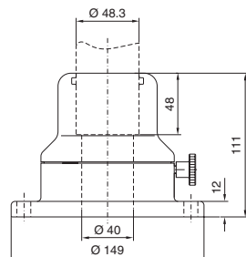
2 Fixation par l'avant CP 6663.400
