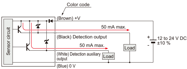
SQ4-A□-P PNP output type
