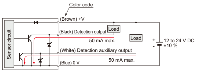
SQ4-A□-N NPN output type
