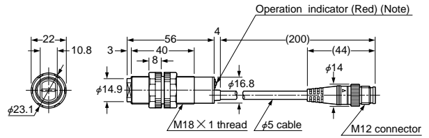
CY-21-J CY-27-J CY-22-J Sensor
