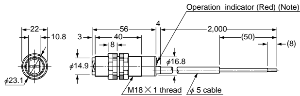
CY-21 CY-27 CY-22 Sensor
