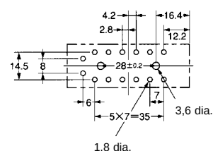
Trous de fixation
