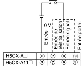
Fonctionne avec relais activé (ON)
