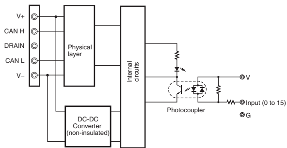
DRT2-ID16ML(X)
