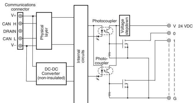
DRT2-MD16 (NPN)
