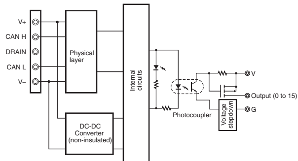
DRT2-OD16ML(X)-1
