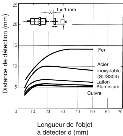
E2E-X14MD
