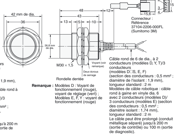
Fig. 16 : E2E-X20MD-F/ E2E-X18ME-F/ E2E-X18MY
