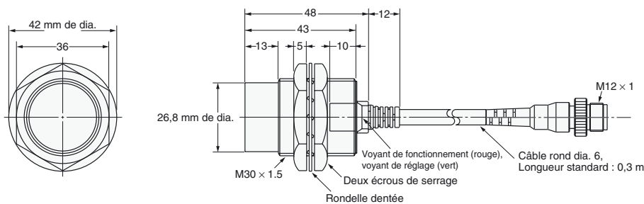
Fig. 35 : E2E-X20MD1-M1GJ
