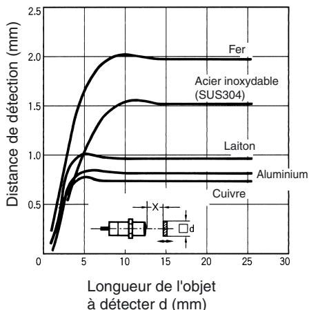
E2E-X2ME□/F□ E2E-X2MY□
