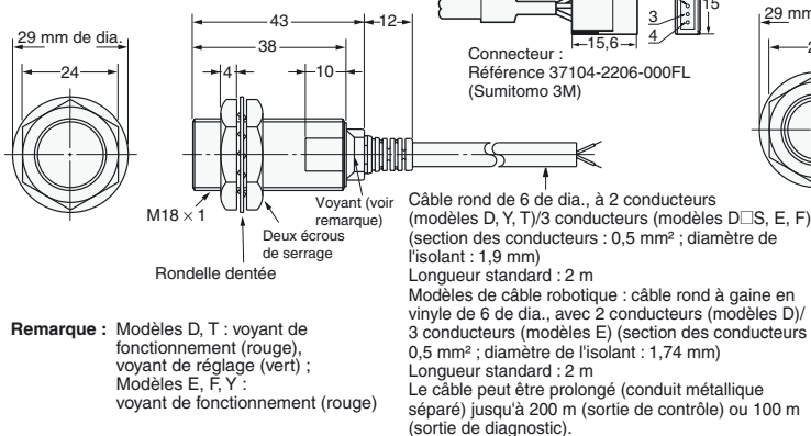
Fig. 13 : E2E-X7D-N/ E2E-X5E-F/ E2E-X5Y-E2E-X7T1
