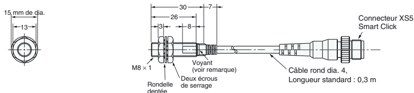
Fig. 30 : E2E-X3D1-M1GJ E2E-X3D1-M1J-T E2E-X3D□-M1TGJ-U
