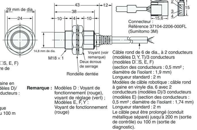
Fig. 16 : E2E-X20MD-F/ E2E-X18ME-F/ E2E-X18MY
