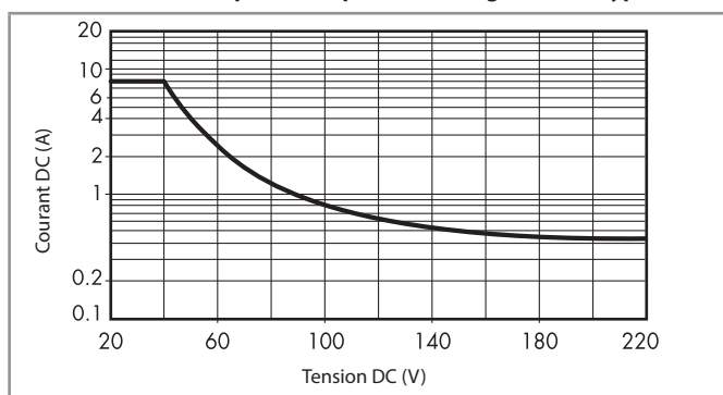
H 50 - Pouvoir de coupure maxi pour une charge en DC1 (type 50.16)
