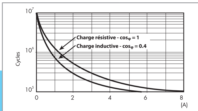
F 50 - Durée de vie électrique (AC) en fonction de la charge (type 50.12)
