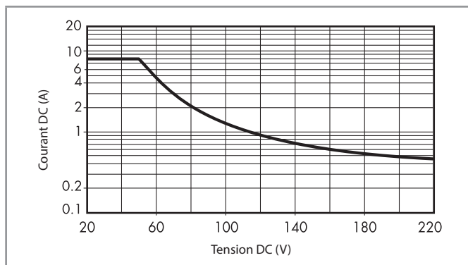
H 50 - Pouvoir de coupure maxi pour une charge en DC1 (type 50.14)
