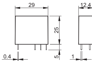
Type 50.12...1000/50.12...5000
