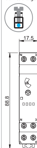
Type 14.71 Bornes à cage
