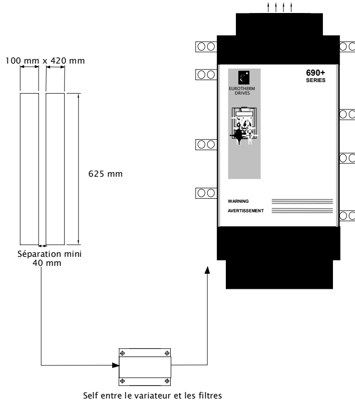
Self entre le variateur et les filtres
