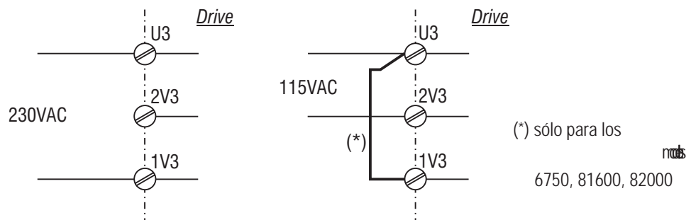
Figura 4.2.3: Conexión externa
