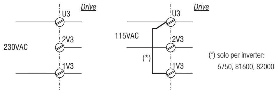
Figura 4.2.3: Collegamento esterno
