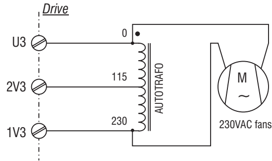
Figure 4.2.1: Connexion de ventilateurs type UL sur les tailles 7900 ... 71320
