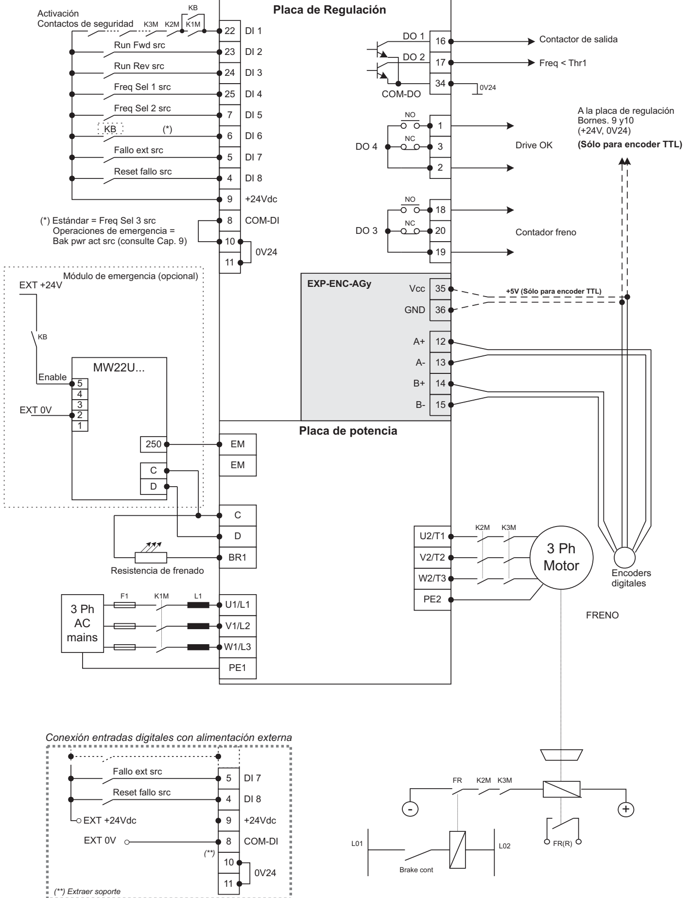
Fig.7.1 – Cableado estándar y conexiones del Módulo de Emergencia MW22U (opcional)
