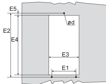
Montaggio con dissipatore esterno Mounting with external dissipator (E)
