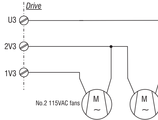
Figure 4.2.1: Connexion de ventilateurs type UL sur les tailles 7900 ... 71320
