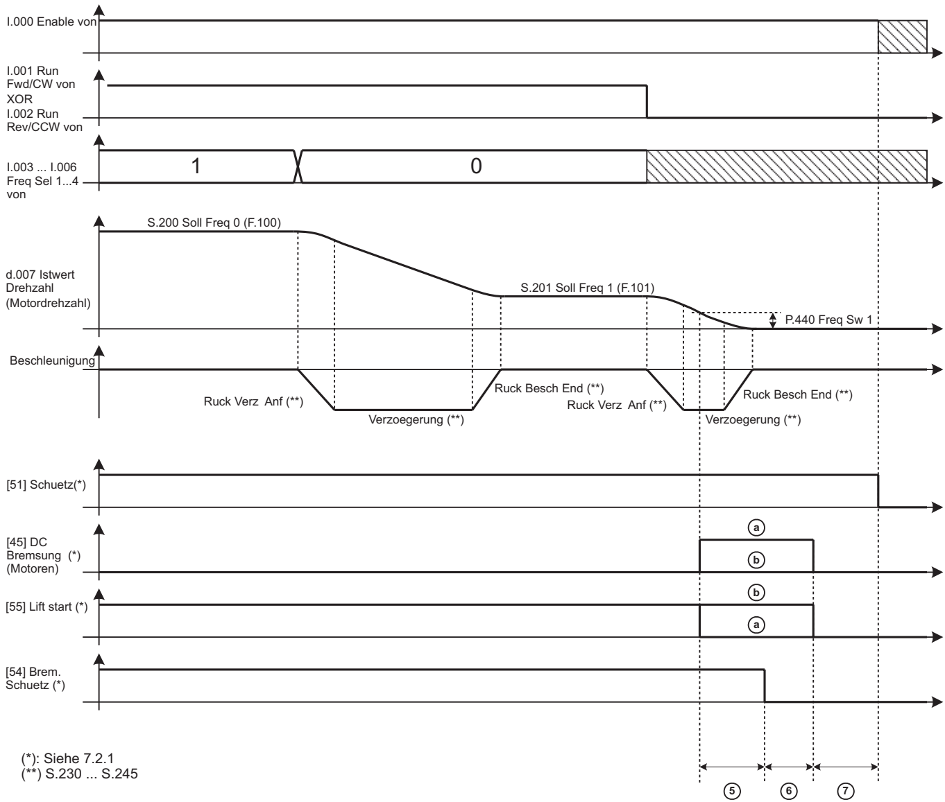
Abb. 7.3 – Detaillierte Haltesequenz
