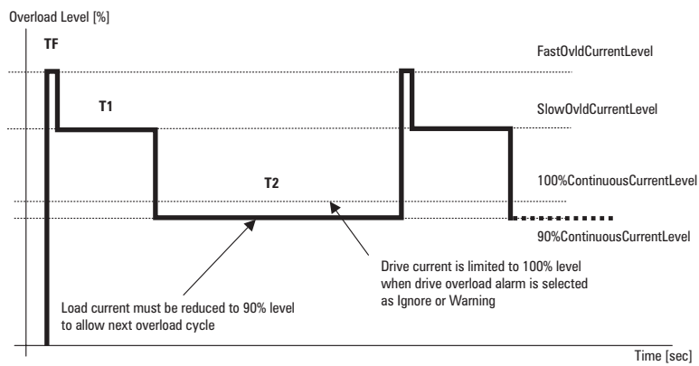
Abbildung 3.5.1-B: Überlastzyklen (Größen 5450... 82000)
