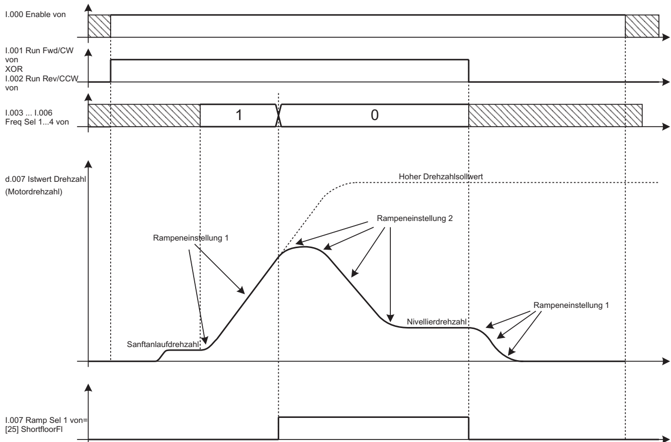
Abb. 7.5 – Kurze Stockwerk-Sequenz
