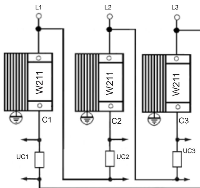
Exemple: montage triangle ouvert pour calibres de 75 à 600 A
