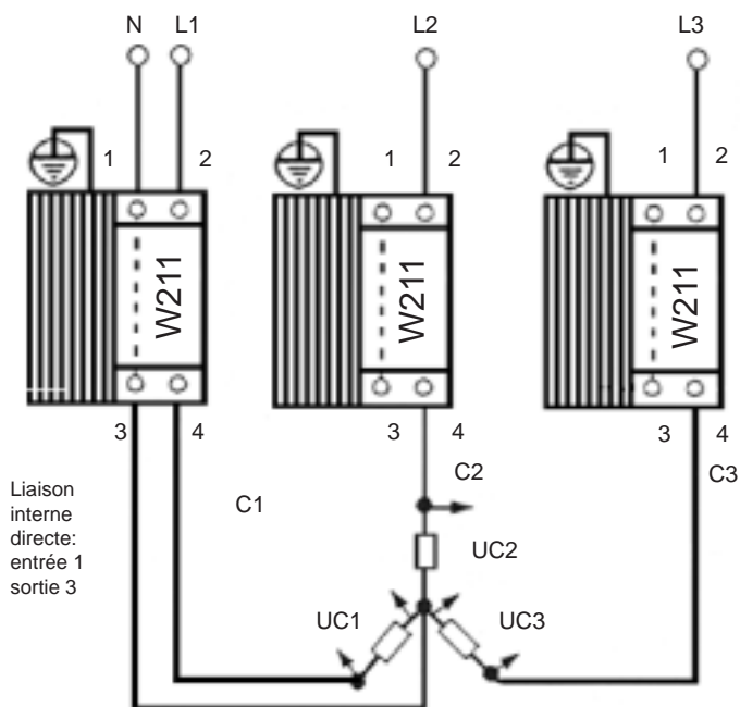
Exemple: montage étoile avec neutre pour calibres 25-40 A
