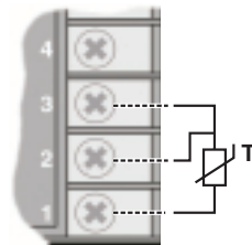
connexion 3 fils
