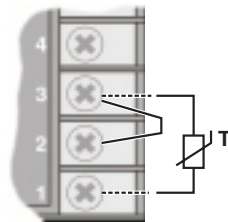
connexion 2 fils
