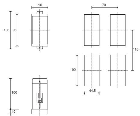
Face avant: 48x96mm (1/8 DIN), profondeur 100mm
