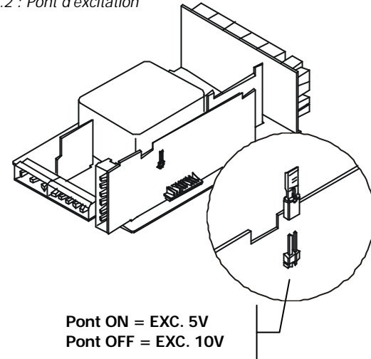
Fig. 18.2 : Pont d'excitation
