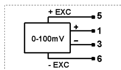
Transducteur 0-100mV
