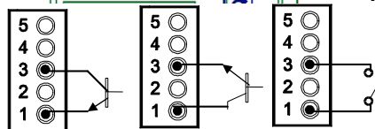
Fig.. 19.2 Exemples de connexion. PNP, NPN ou par contact sec.
