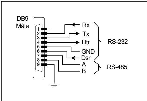
Raccordement série DN-109X , DN-119X et DN-129X
