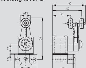
// Drehhebel D Rocking lever D
