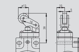
// Drehhebel D Rocking lever D
