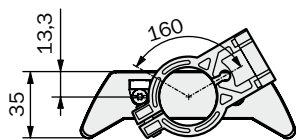
Fixation orientable à rotule (réf. 2019659)
