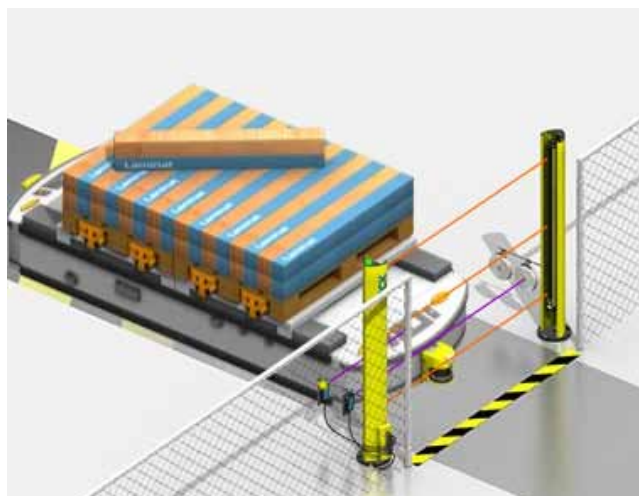
Surveillance de sortie des matériaux avec 2 capteurs d'inhibition dans la zone dangereuse, flux des matériaux vers l'extérieur de la zone dangereuse
