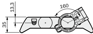
Fixation orientable à rotule (réf. 2019659)
