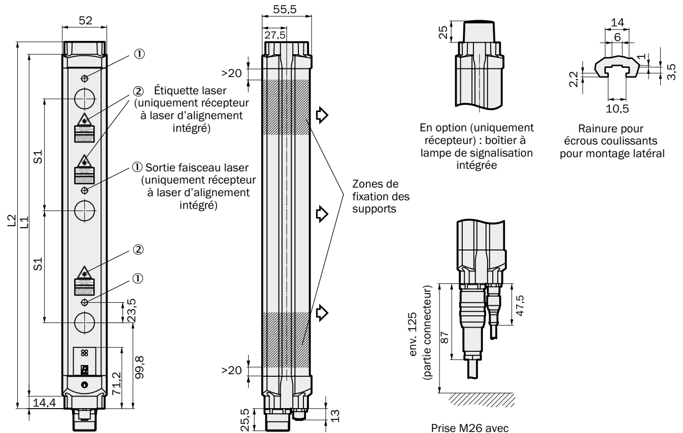
M4000 Advanced (récepteur) ou M4000 Advanced A/P
