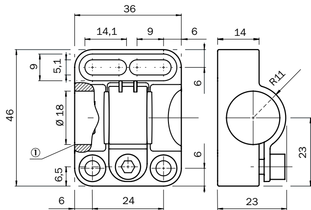
① Sans butée fixe
