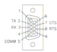
RS-232 DB9-F
