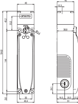
Interrupteur FY 6••D6D•• Principe de fonctionnement D avec déverrouillage auxiliaire à serrure et bouton de déverrouillage antipanique
