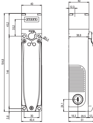
Interrupteur FY 6••D7D•• Principe de fonctionnement D avec déverrouillage auxiliaire plombable et bouton de déverrouillage antipanique
