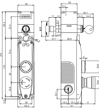
Interrupteur FY 6•••••••• avec dispositifs de commande intégrés
