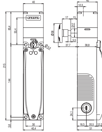
Actionneur VF KEYF21
