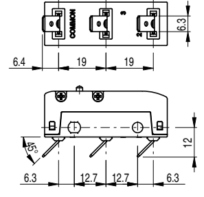
Bornes à faston G , pli gauche (sur demande)
