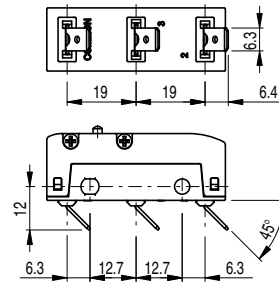
Bornes à faston F , pli droite
