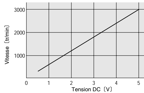
Rapport entre la vitesse et la tension DC appliquée. (Valeur indicatives).
