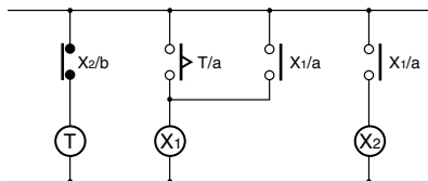
⊗ : Relais auxiliaires de type G2R
