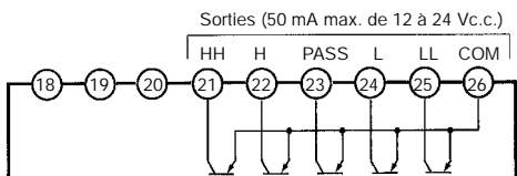
K31-L1, L2, L3, -L4, -L5, -L6, -L7, -L8, -L9, -L10 : Linéaire (Les bornes 21 à 26 existent uniquement sur les K31-L4, -L5, -L6, -L9, -L10.)
