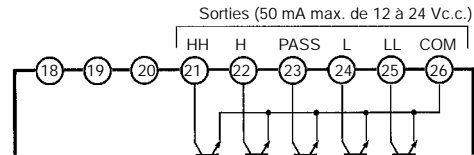
K31-T1 : Transistor (collecteur NPN ouvert)
