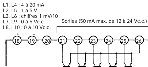
K31-L1, L2, L3, -L4, -L5, -L6, -L7, -L8, -L9, -L10 : Linéaire (Les bornes 21 à 26 existent uniquement sur les K31-L4, -L5, -L6, -L9, -L10.)
