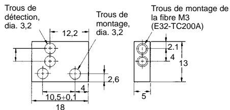
E39-F5 Kit de conversion pour réflexion diffuse latérale
