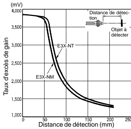
E32-CC200
