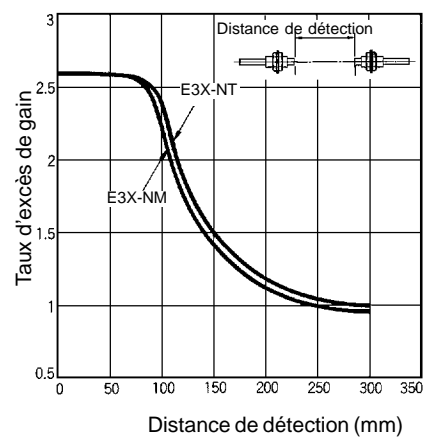
E32-T16
