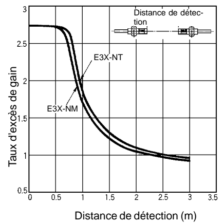
E32-T21L
