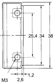
Réflecteur (bande) E39-RSA (à commander séparément)
