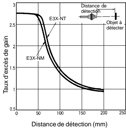
E32-DC200
