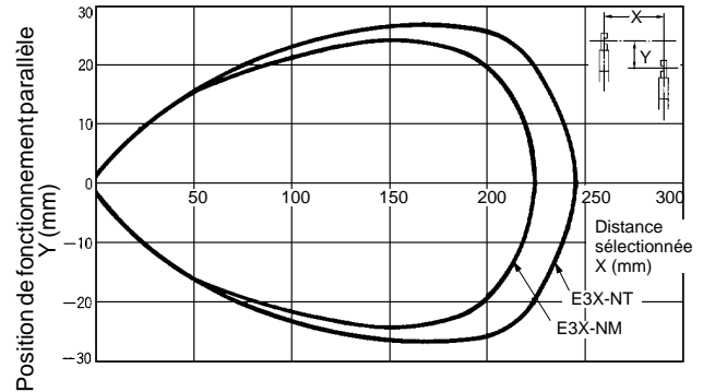
E32-T12F
