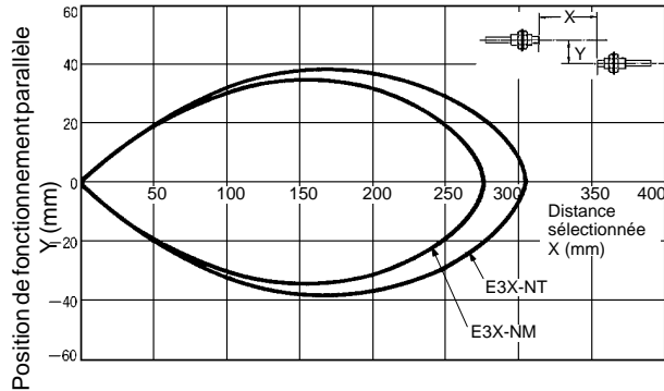
E32-T17L
