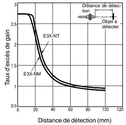
E32-D21L
