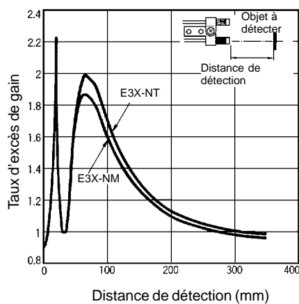
E32-T17L
