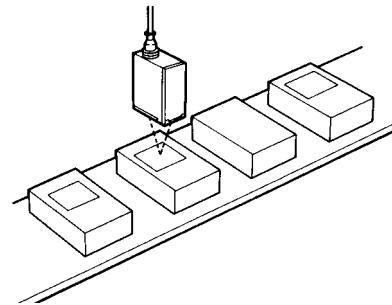
Détection d'étiquettes
