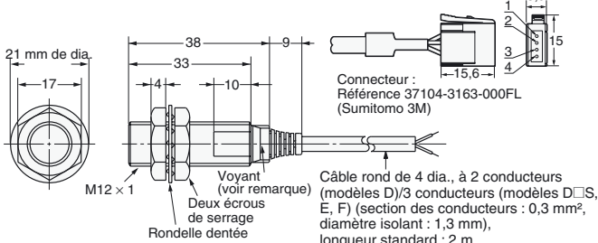
Fig. 8 : E2E-X3D□-N E2E-X2E□/F□
