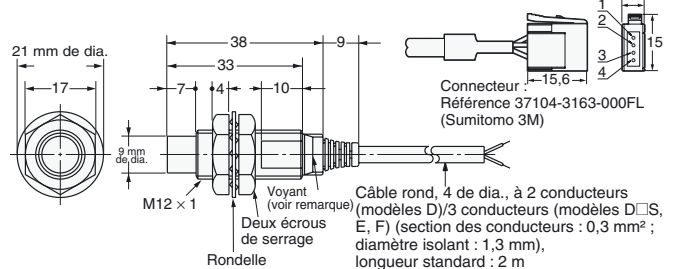
Fig. 9 : E2E-X8MD□ E2E-X5ME□/F□
