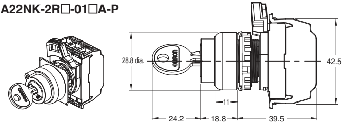
A22NK-2R□-01□A-P
