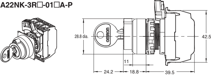
A22NK-3R□-01□A-P
