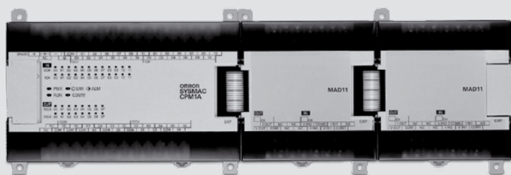
UC CPM2A avec deux cartes E/S analogiques CPM1A-MAD11 (2 entrées et 1 sortie analogiques)
