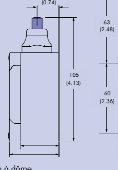
Boîtiers en Métal 440P-M 30MM
