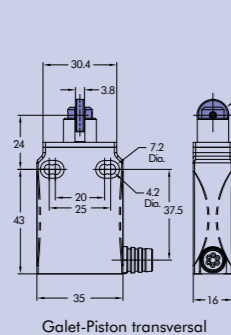
Boîtiers en Métal Compact 440P-A
