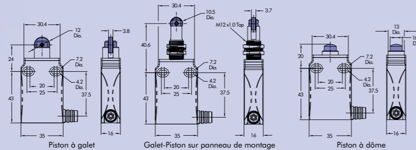
Dimensions approximatives - en mm (pouces)
