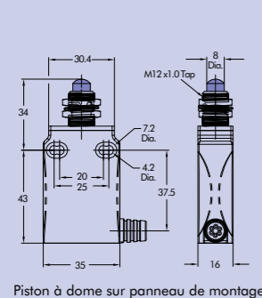
Dimensions approximatives - en mm (pouces)
