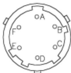
Connecteur 6 broches PT06A-10-6S
