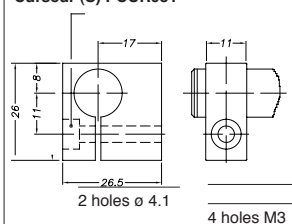
Curseur (S) PCUR031
