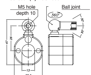
Curseur (B) PCUR033
