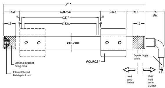
Version PME12 C sortie connecteur
