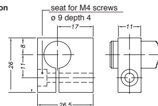
Curseur (B) PCUR033
