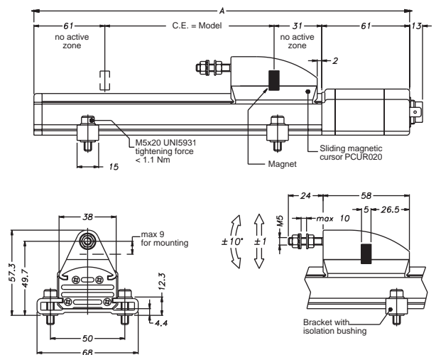
Version MK2C F avec curseur magnétique flottant
