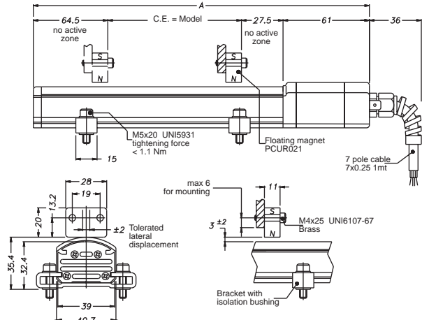
Version MK2C F avec curseur magnétique flottant
