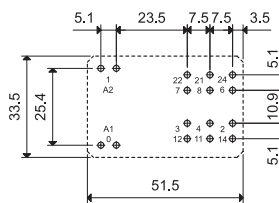
Vue coté cuivre
