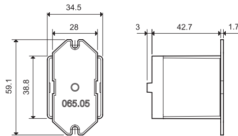
Adaptateur avec patte sur le dessus, pour types 65.31.xxxx.xxx9
