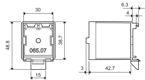
Adaptateur rail 35 mm (EN 60715) sur le dessus pour types 65.31.xxxx.xxx9
