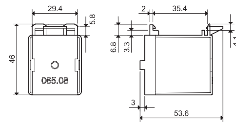
Adaptateur rail 35 mm (EN 60715) à l'arrière pour types 65.31.xxxx.xxx9
