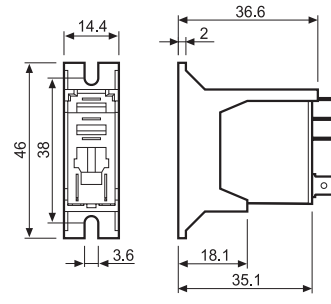
046.05 avec relais monté
