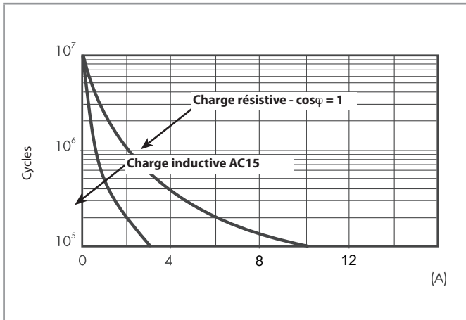
F 40.6 - Durée de vie électrique (AC) en fonction de la charge Type 40.62
