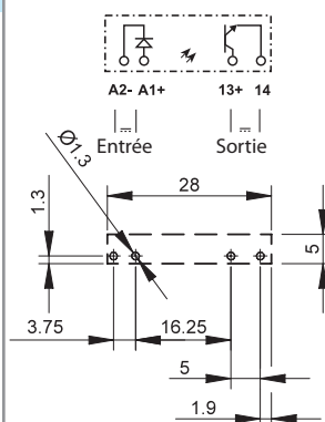
Vue coté cuivre
