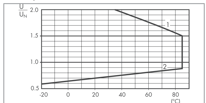
R 34 - Plage de fonctionnement bobine DC en fonction de la température ambiante
