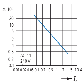
Longévité de l'appareil (manœuvres)
