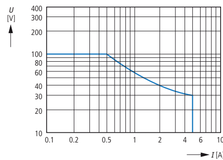
Charge DC (ohmique)
