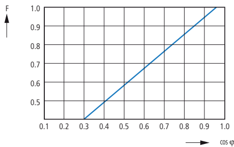
Facteur de réduction pour charge inductive AC
